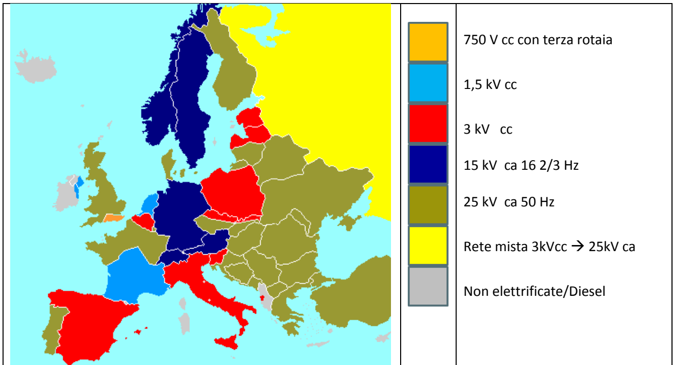
Fig. 2 – Sistemi di alimentazione elettrica di trazione utilizzati in Europa
