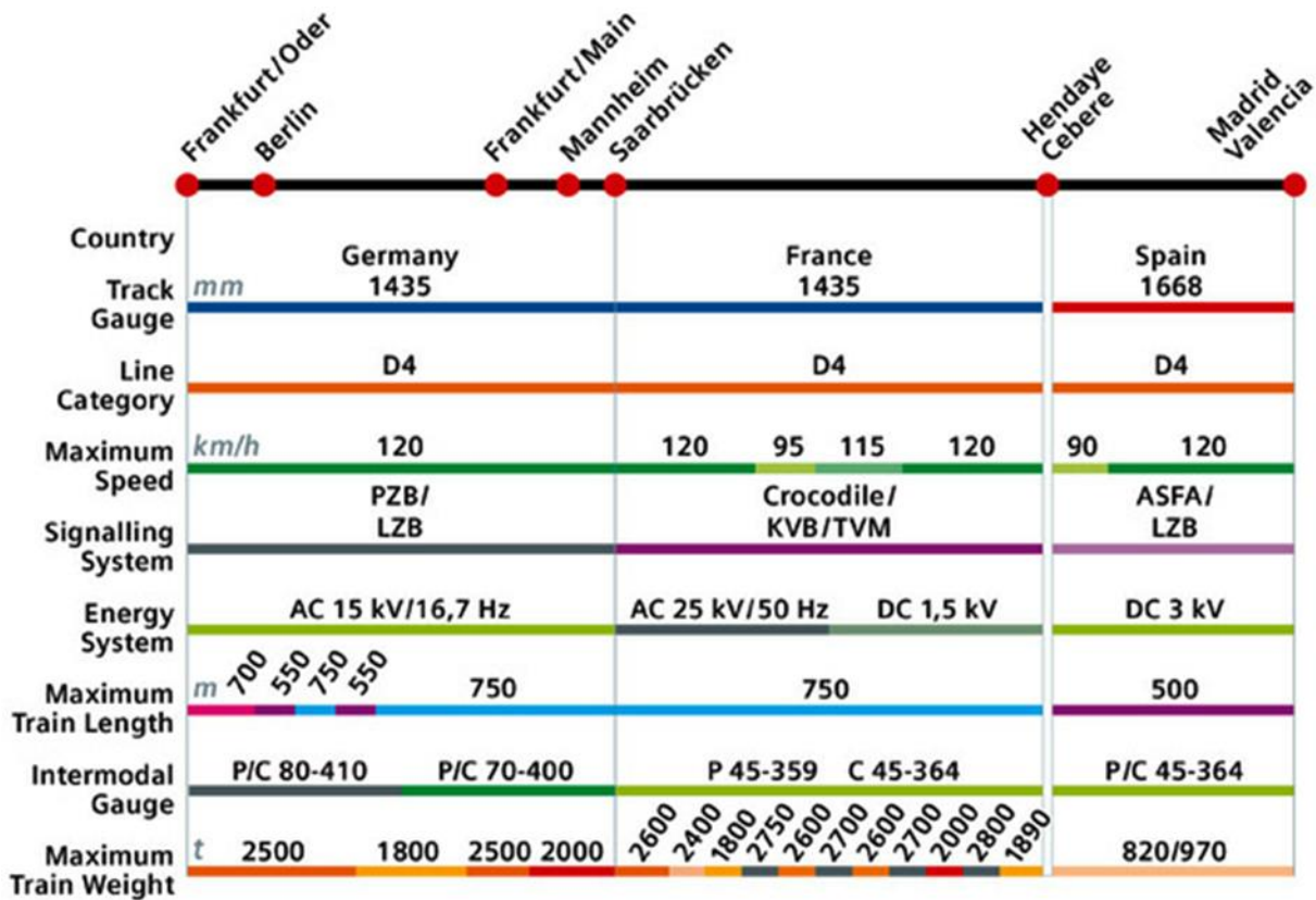
Fig. 4 - Esempio di ostacoli tecnici che un treno deve superare tra Francoforte / Oder a Madrid
