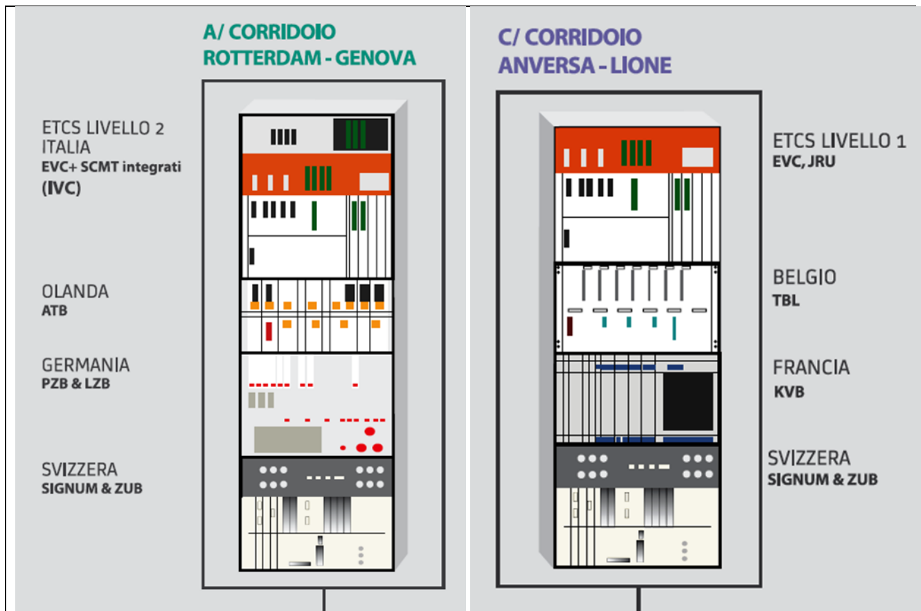
Fig. 6 - Apparecchiature di segnalamento a bordo di un locomotore per due specifici corridoi
