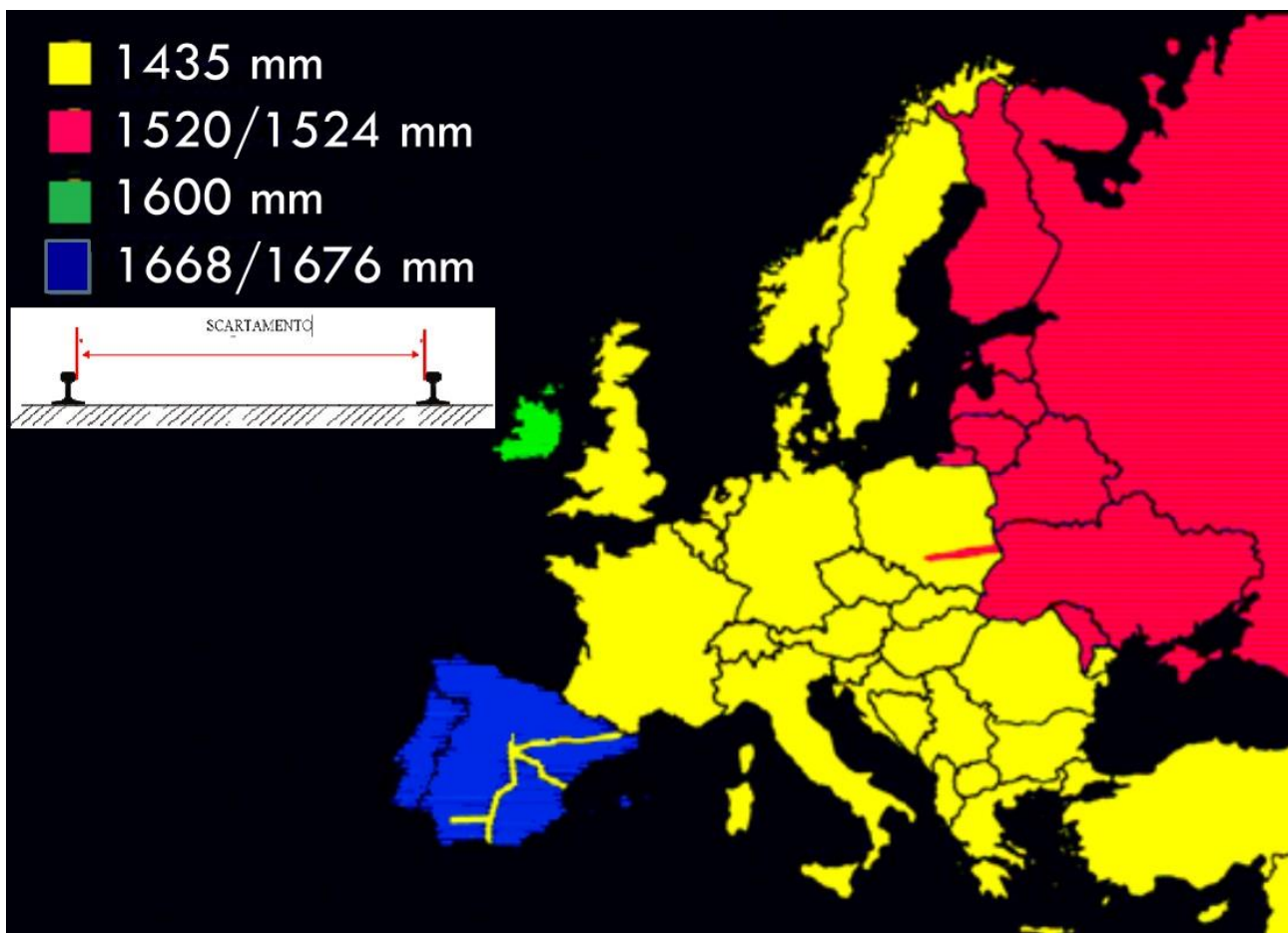
Fig. 1 – Scartamenti ferroviari utilizzati in Europa
