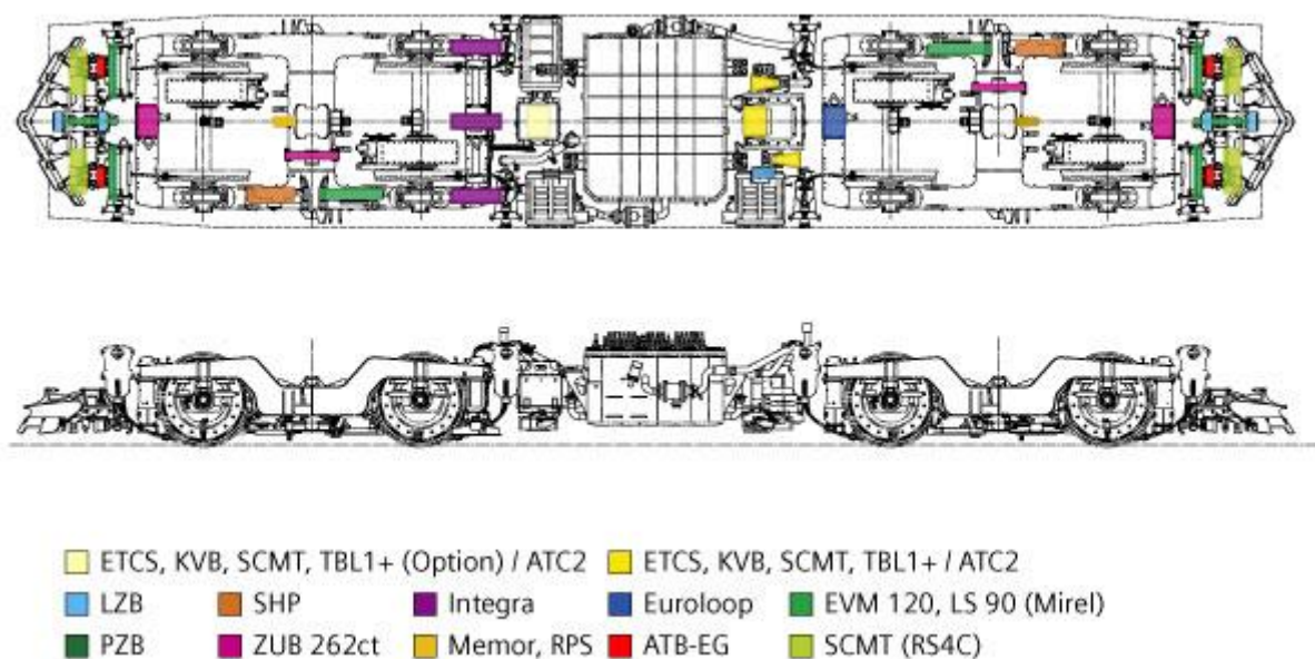
Fig. 5 - Locomotore con componenti interoperabili modulari
